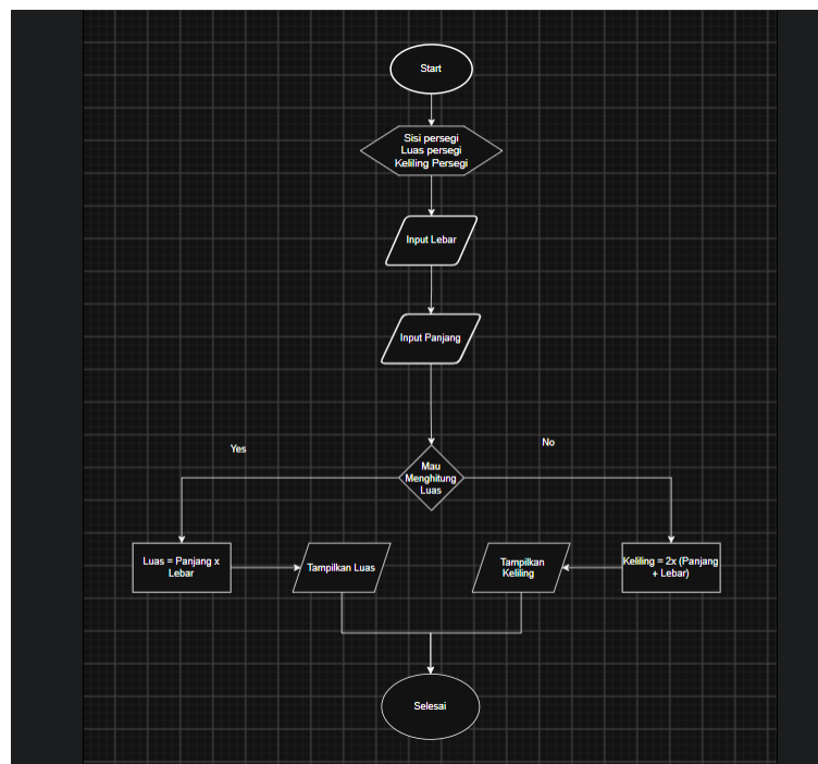
Gambar 1.1 Flowchart menghitung rumus luas dan keliling persegi panjang
